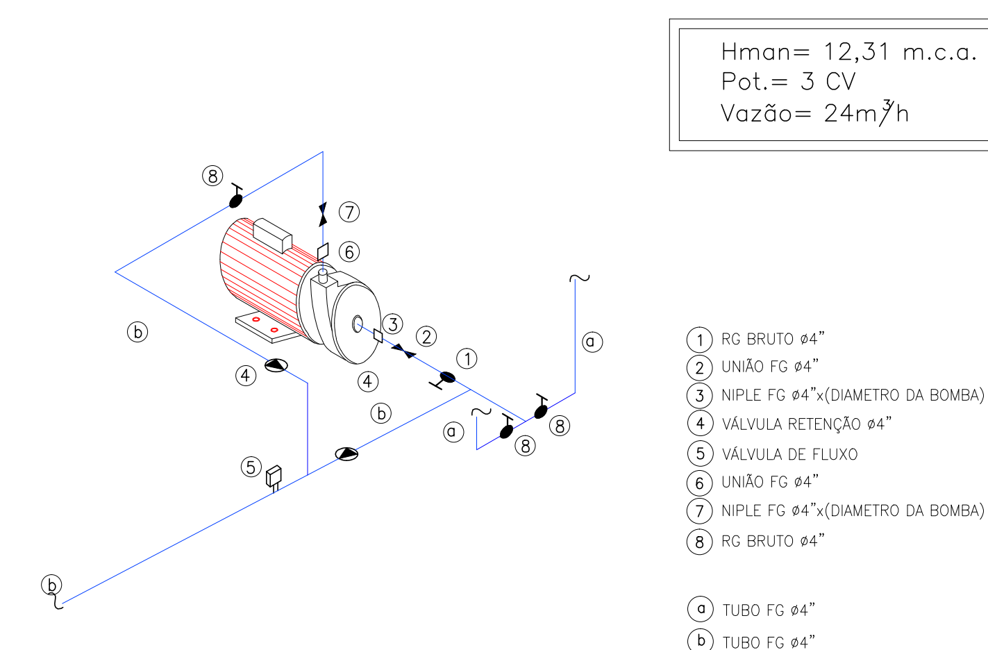
DETALHE DA BOMBA DE INCÊNDIO ESQ. 14/98
