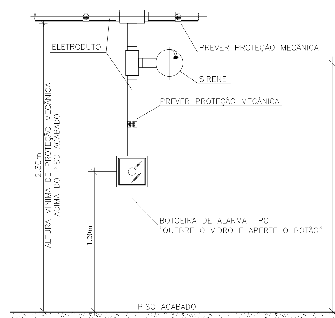
SIRENE E ACIONADOR MANUAL (BOTOEIRA)
